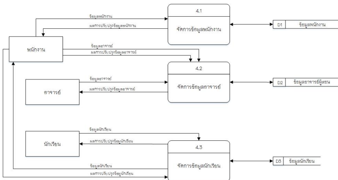
ภาพที่ 3.8 แผนภาพกระแสข้อมูล DFD Level 1 โปรเซสที่ 4 จัดการข้อมูลผู้ใช้ระบบ
